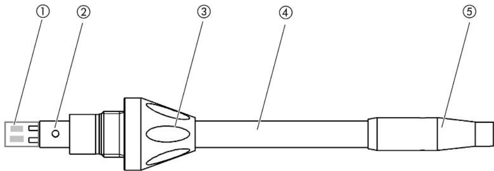
插图 7: 探尖
