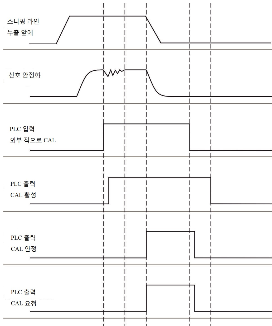
약어 6: 스니퍼 라인 SL3000XL의 예시에서 IO1000을 통한 외부 보정, PLC 입력부 및 출력부 묘사: "입력부 및 출력부 할당 [▶ 56]" 참조
