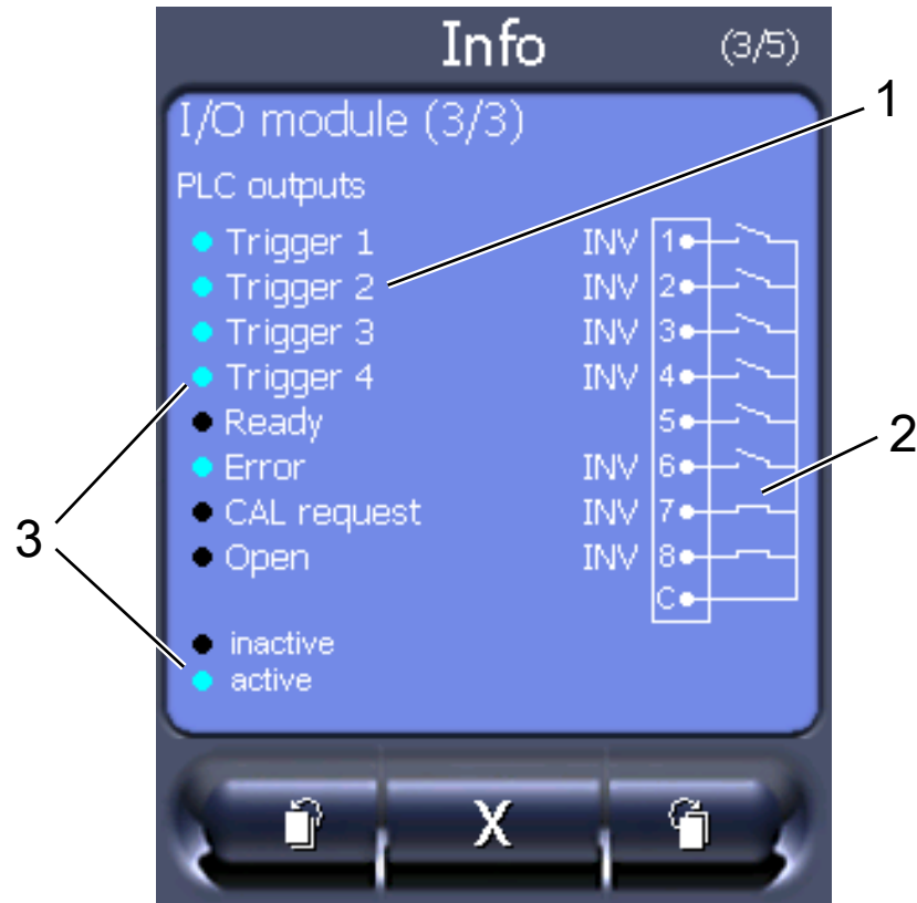
약어 13: 디지털 출력부 관련 시각화 정보
