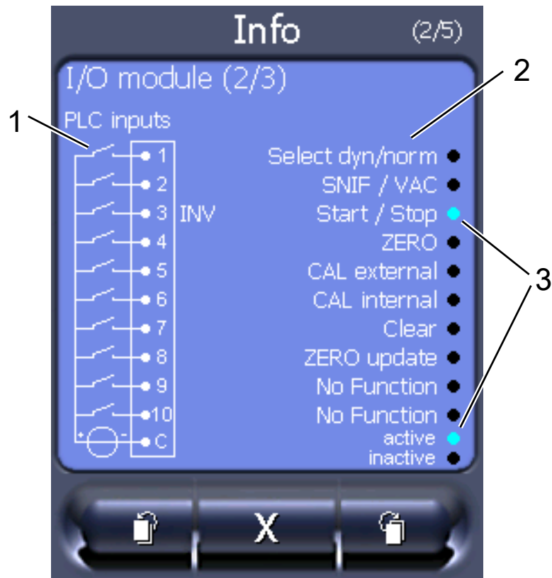
약어 12: I/O 모듈(2): 디지털 입력부 관련 시각화 정보
