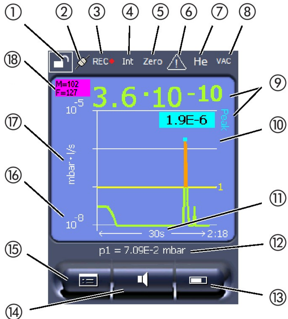
약어 11: 측정 디스플레이
