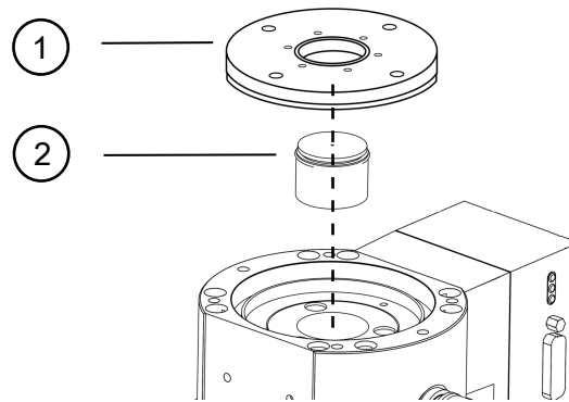
1 커버 플레이트
