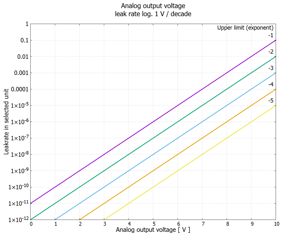
약어 9: 아날로그 출력 전압 누설률 대수 1 V/디케이드
