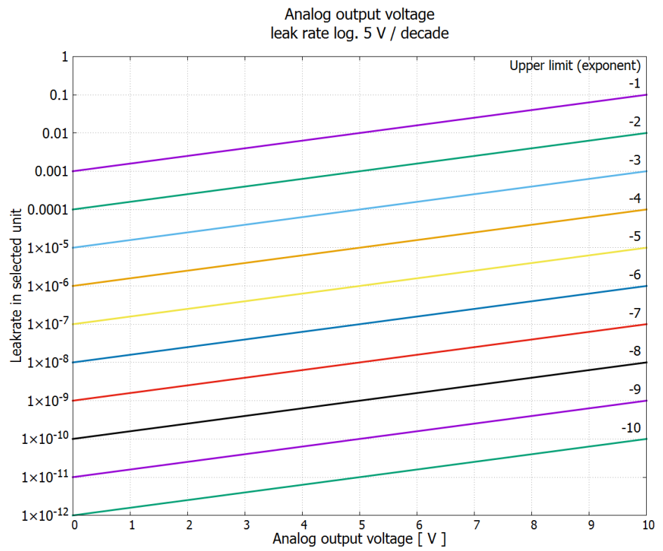
약어 10: 아날로그 출력 전압 누설률 대수 5 V/디케이드
