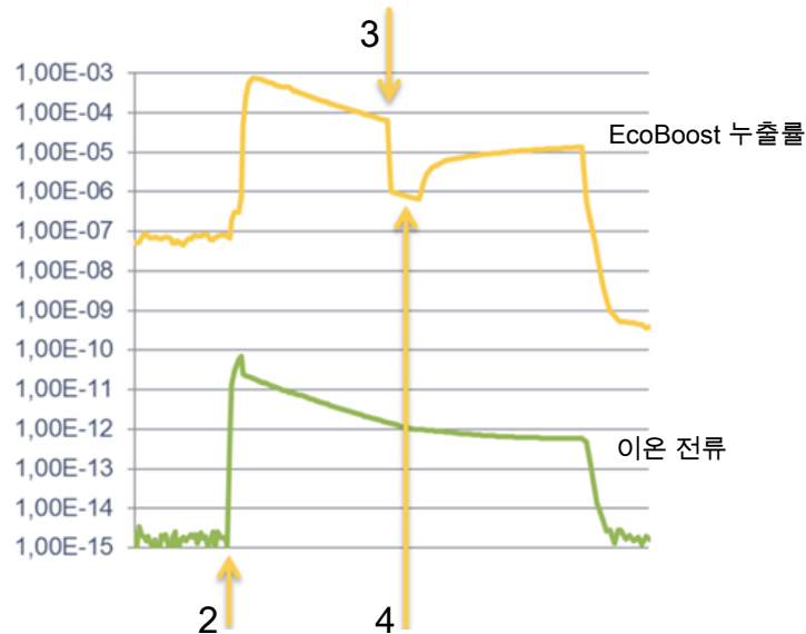
약어 8: 측정 곡선 예시(EcoBoost)
