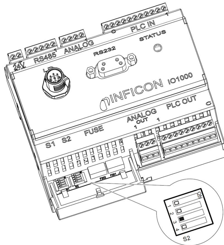
약어 16: I/O 모듈 DIP 스위치
