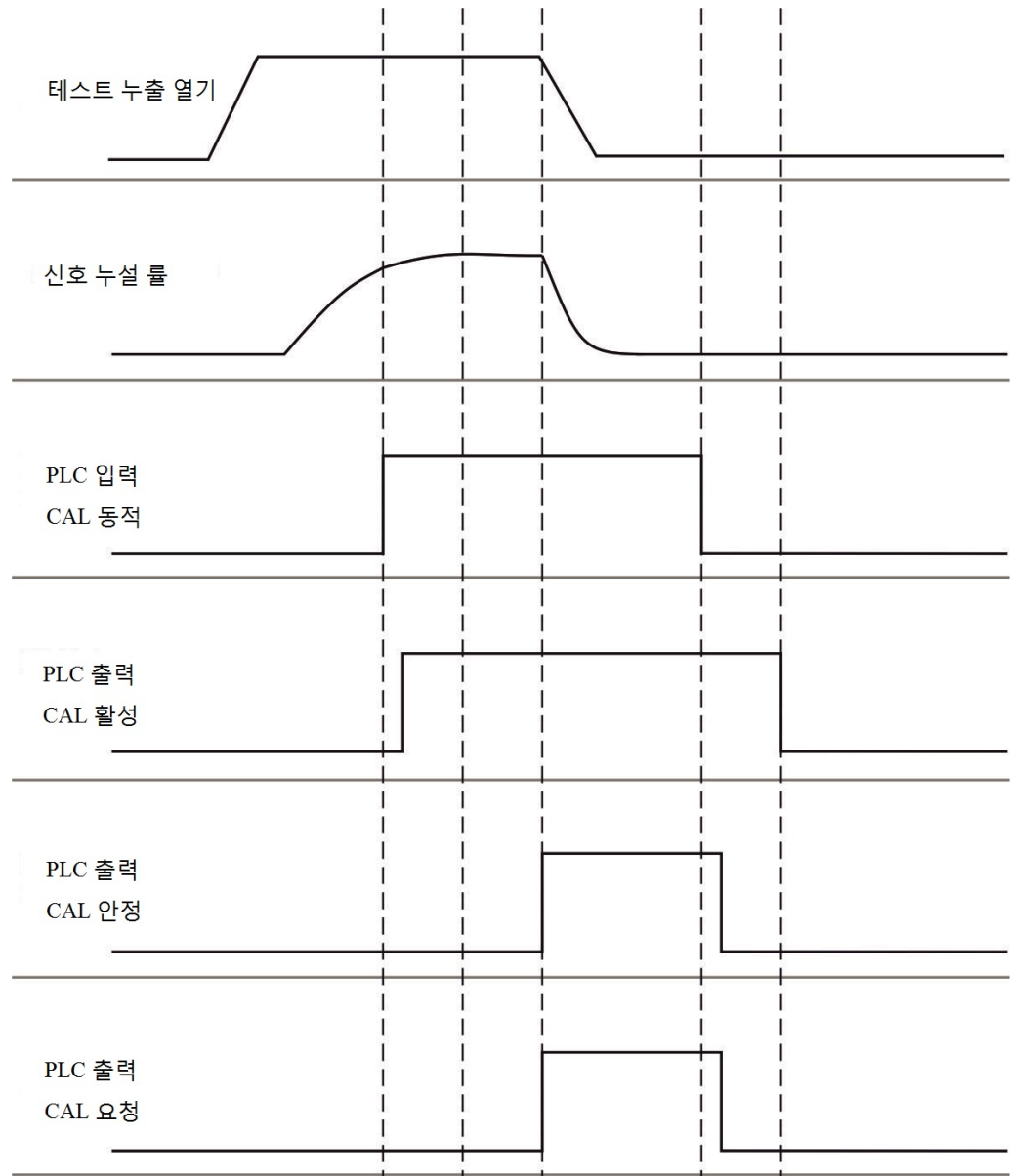
약어 7: 그림 7 스니퍼 라인 SL3000XL의 예시에서 IO1000을 통한 외부 동적 보정, PLC 입력 및 출력부 설명: "입력부 및 출력부 할당 [▶ 56]" 참조
