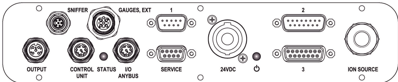
약어 3: MSB 박스 연결부
