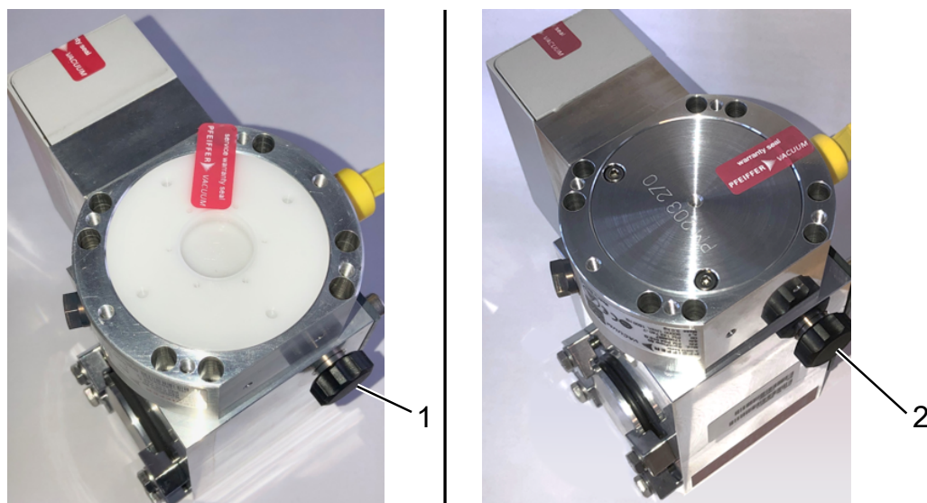
図 17: カバーが異なるターボ分子ポンプSplitFlow 80
