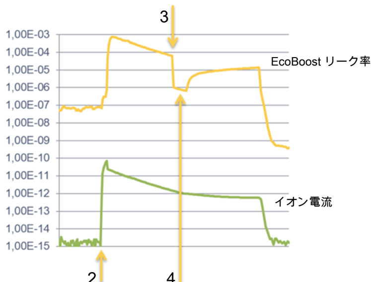
図 8: 測定曲線例 (EcoBoost)
