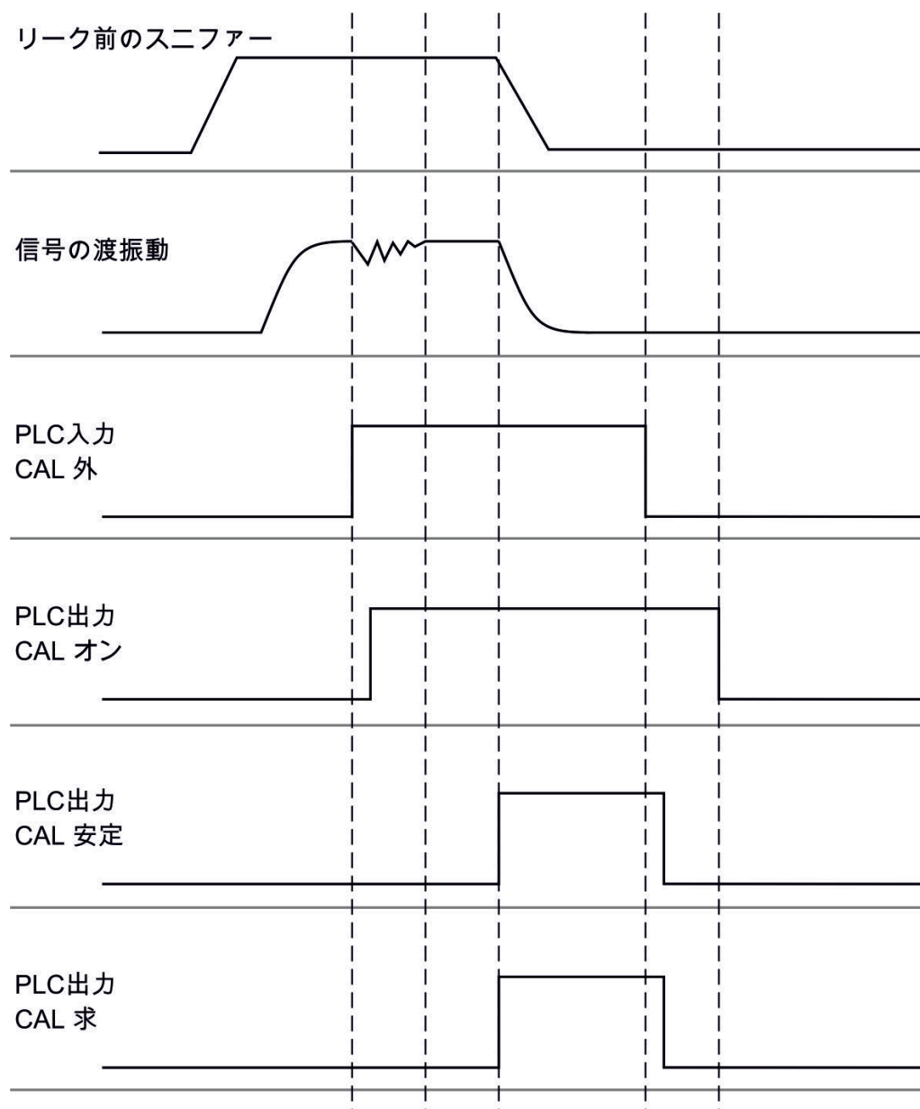
図 6: 例として、スニファーラインSL3000XLを使用した際のIO1000における外部校正。PLC入出力の説明：「入出力の割り当て [▶ 59]」を参照
