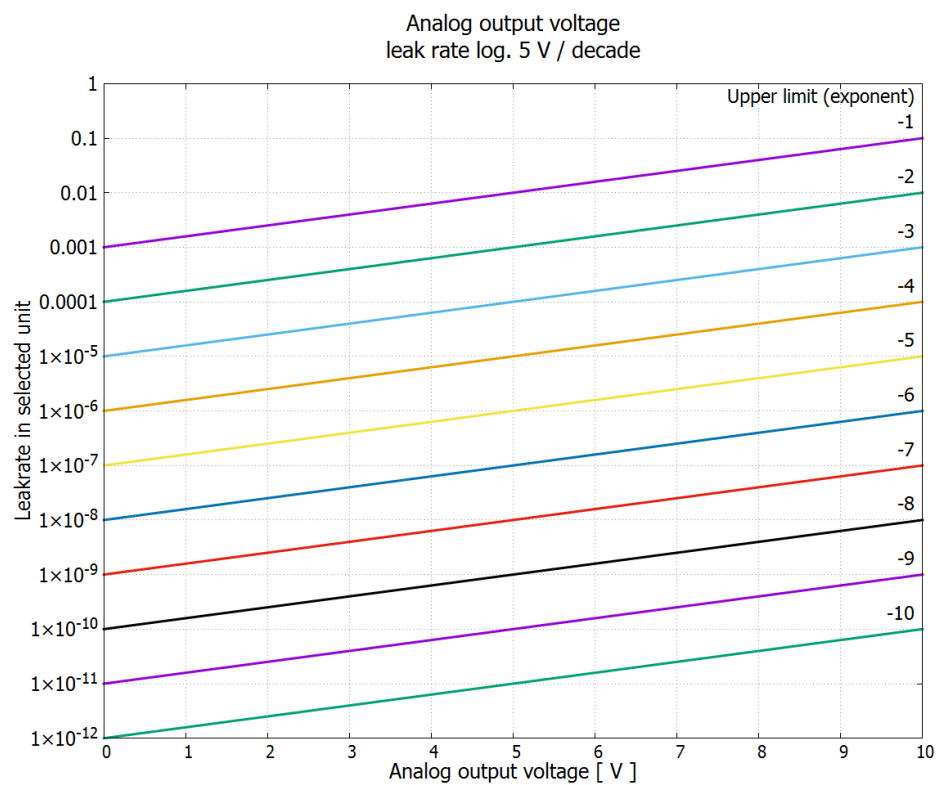
図 10: アナログ出力電圧リークレート対数 5 V/decade
