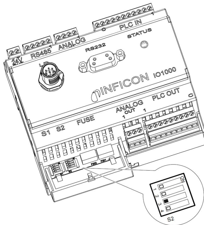
図 16: I/OモジュールのDIPスイッチ
