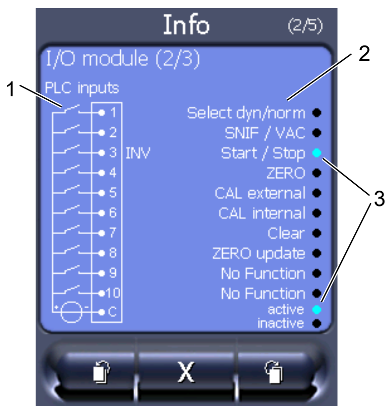
図 12: I/O モジュール (2)：デジタル入力に関する情報のグラフ表示
