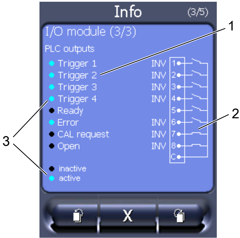
図 13: デジタル出力に関する情報のグラフ表示
