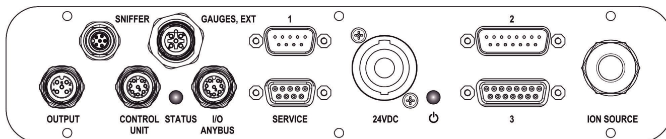
図 3: MSBボックス接続部
