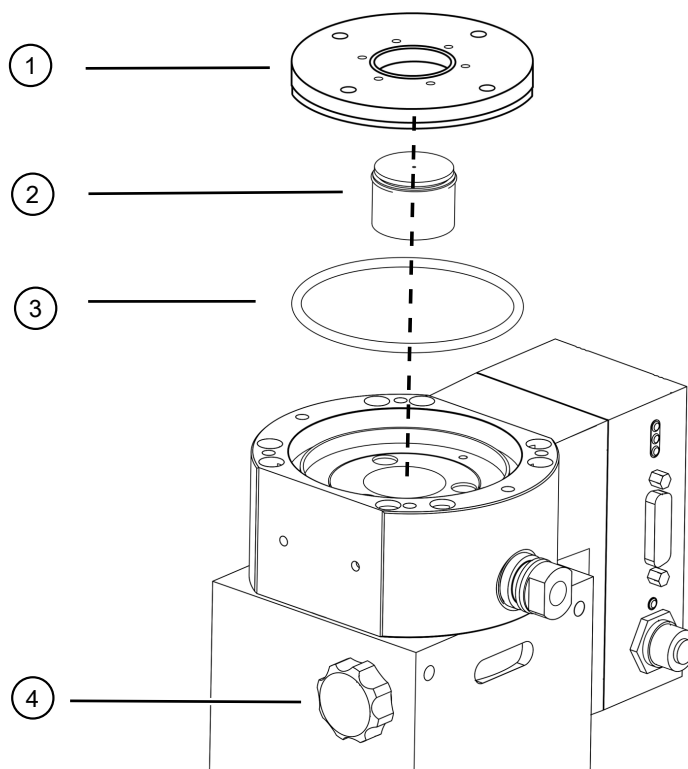
図 19: 図はモデルAを示しています
