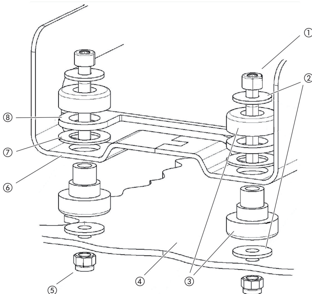
図 5: 留め具の構成
