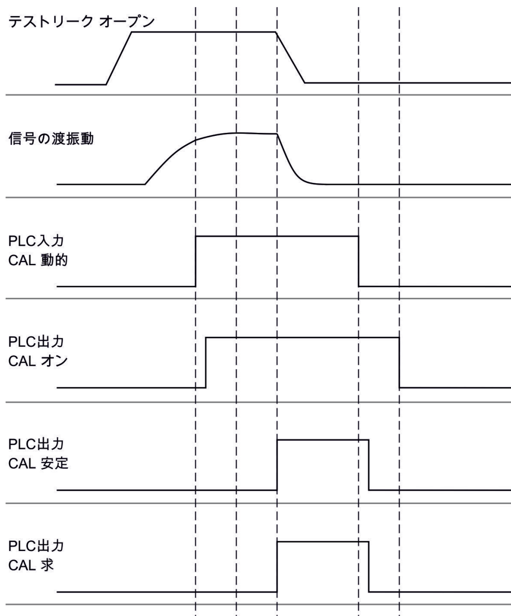
図 7: 図 7 例としてスニファーマーラインSL3000XLを使用した際のIO1000における外部動的校正。 PLC入出力の説明: 「入出力の割り当て [▶ 59]」を参照
