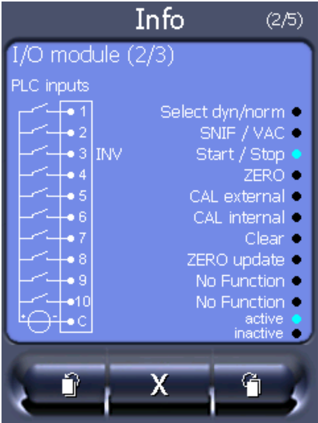
Рис. 7: Модуль I/O (2): Визуализированная информация о цифровых входах
