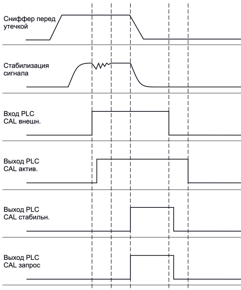
Рис. 5: Внешняя калибровка с IO1000 на примере детекторной линии SL3000XL, описание входов и выходов ПЛК: см. Занятие аналоговых выходов модуля I/O [► 49]
