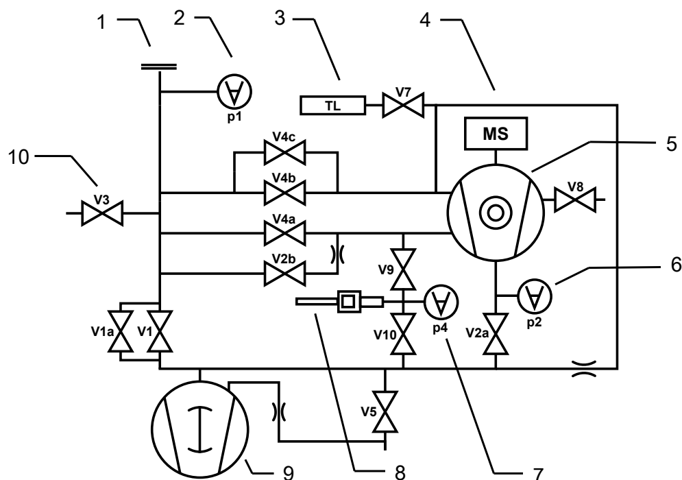
Рис. 14: Основные компоненты диаграммы вакуума в приборах UL3000 Fab ULTRA
