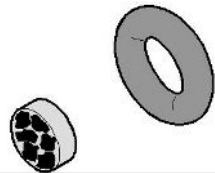
Рис. 17: На металлокерамическом фильтре сильные загрязнения
