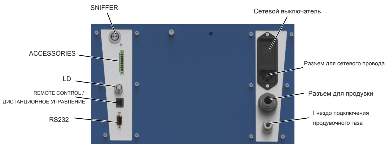
Рис. 6: Подключения принадлежностей и управляющих сигналов
