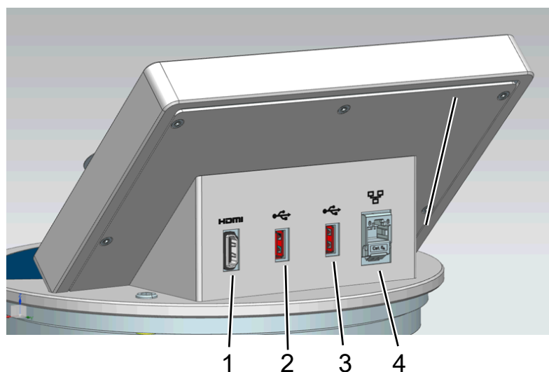
Рис. 5: Блок управления (вид сзади)
