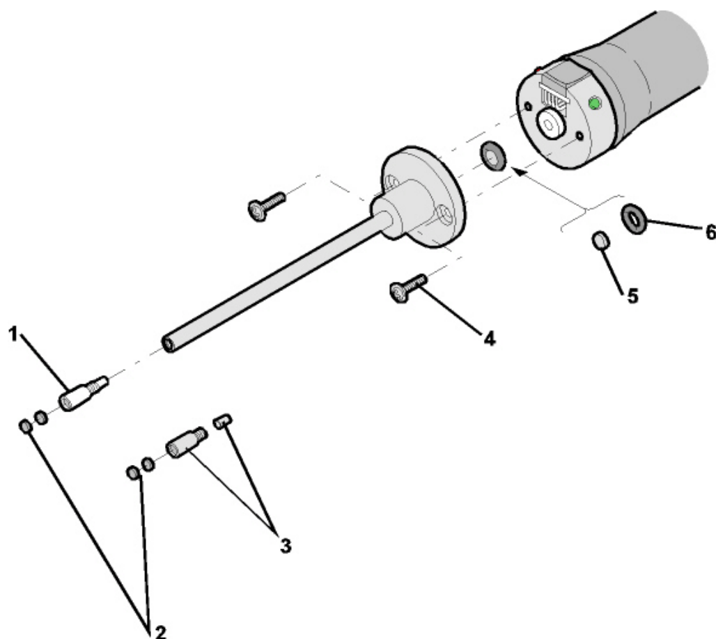
Рис. 15: Детекторный наконечник
