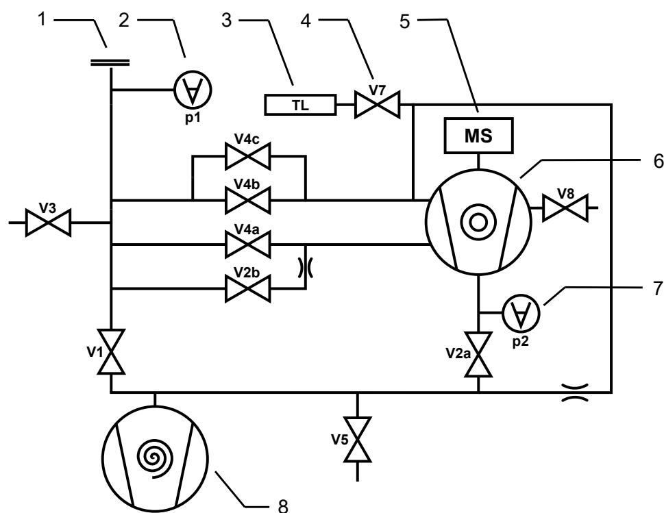
Fig. 14: UL3000 Fab : Principaux composants du diagramme du vide
