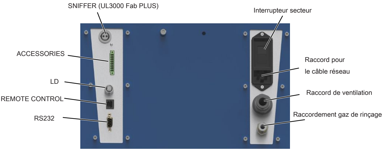
Fig. 6: Raccords pour accessoires et signaux de commande
