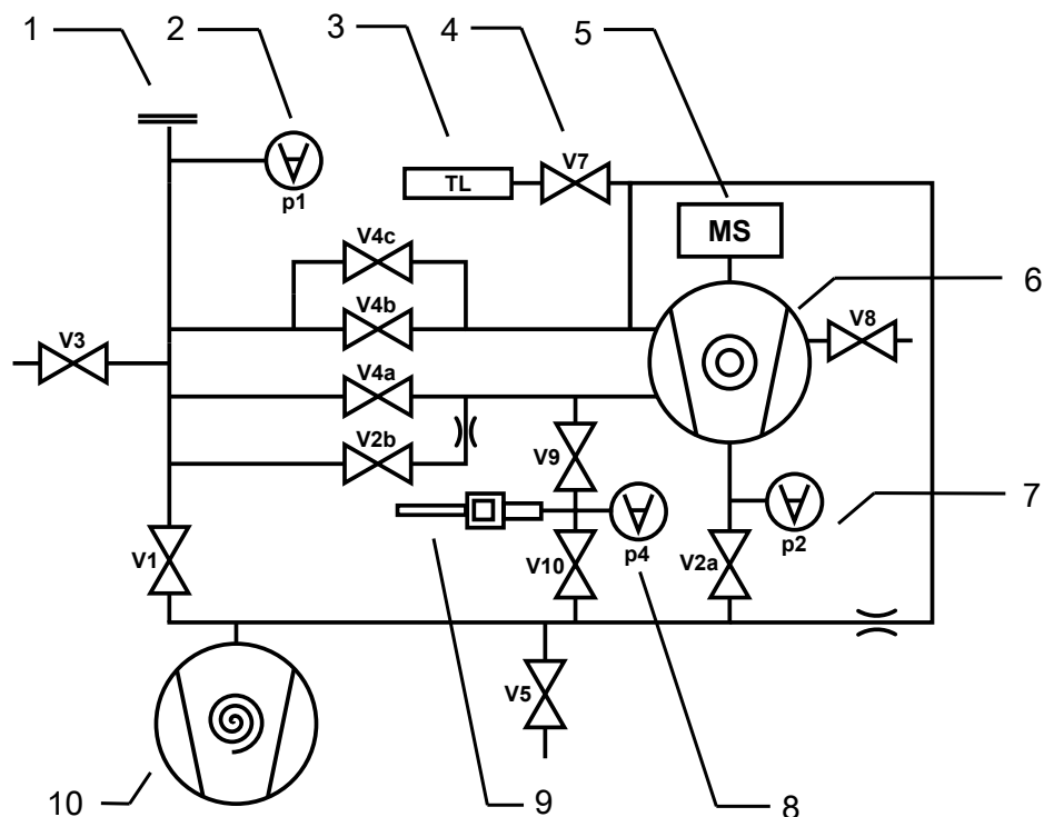
Fig. 15: UL3000 Fab PLUS : Principaux composants du diagramme du vide
