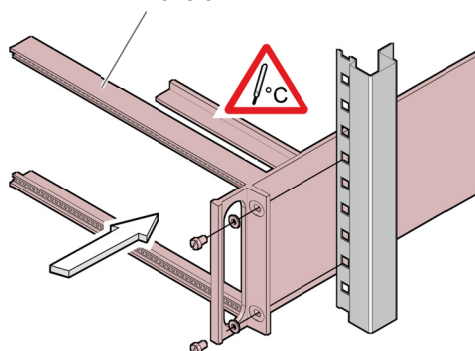
Rackeinschubadapter Höhe 3
