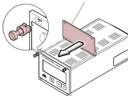
Rackeinschubadapter Höhe 2 zu Höhe 3
