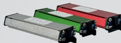
De gauche à droite : capteur de fluide frigorigère 724-701-G1, capteur de CO 2 724-701-G2 et capteur de fluide frigorigère inflammable 724-701-G3.
