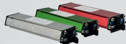
Von links nach rechts: Kältemittelsensor 724-701-G1, CO 2 -Sensor 724-701-G2 und Sensor für brennbare Kältemittel 724-701-G3.
