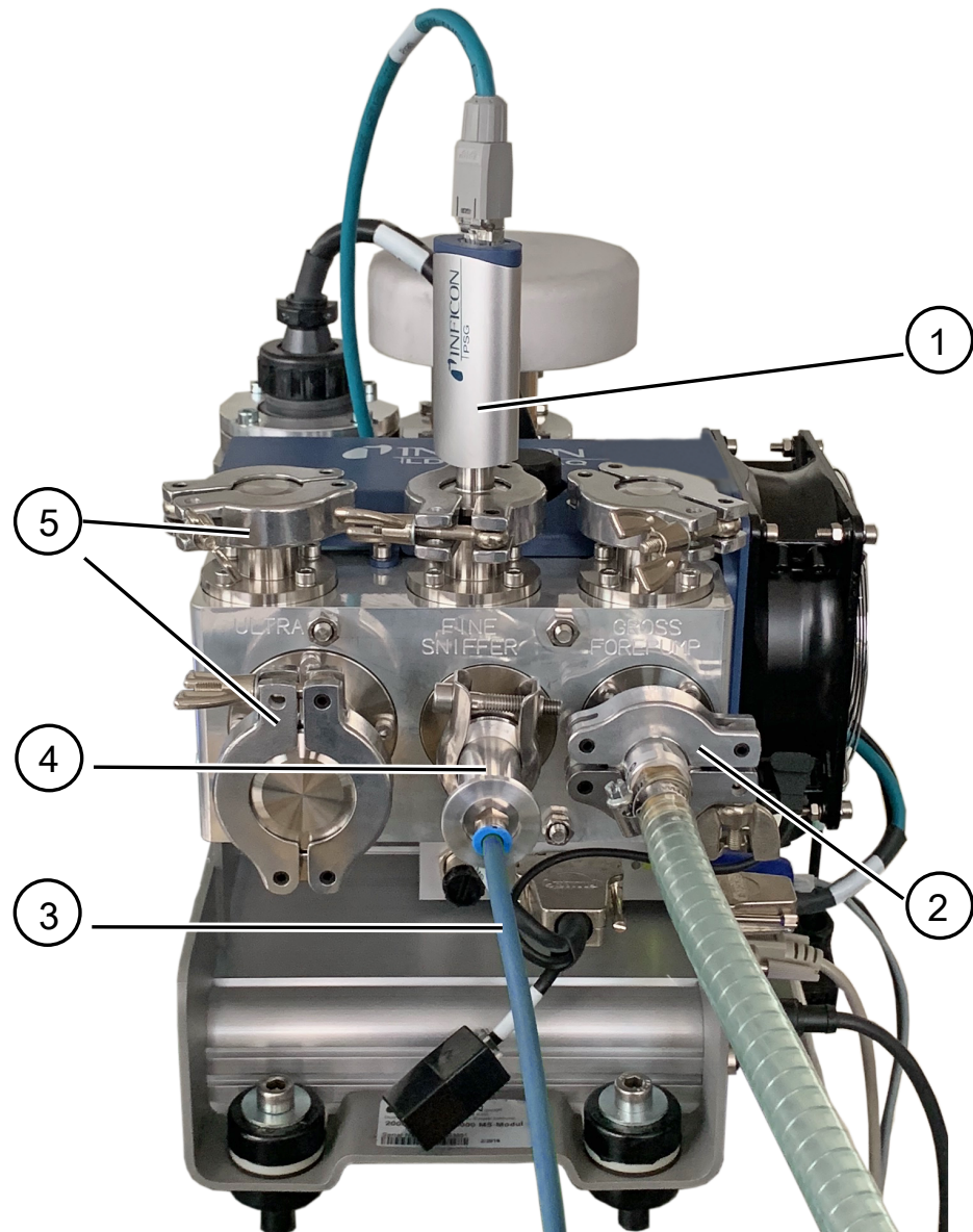
약어 2: 질량 분석기 모듈(측정 사양)
