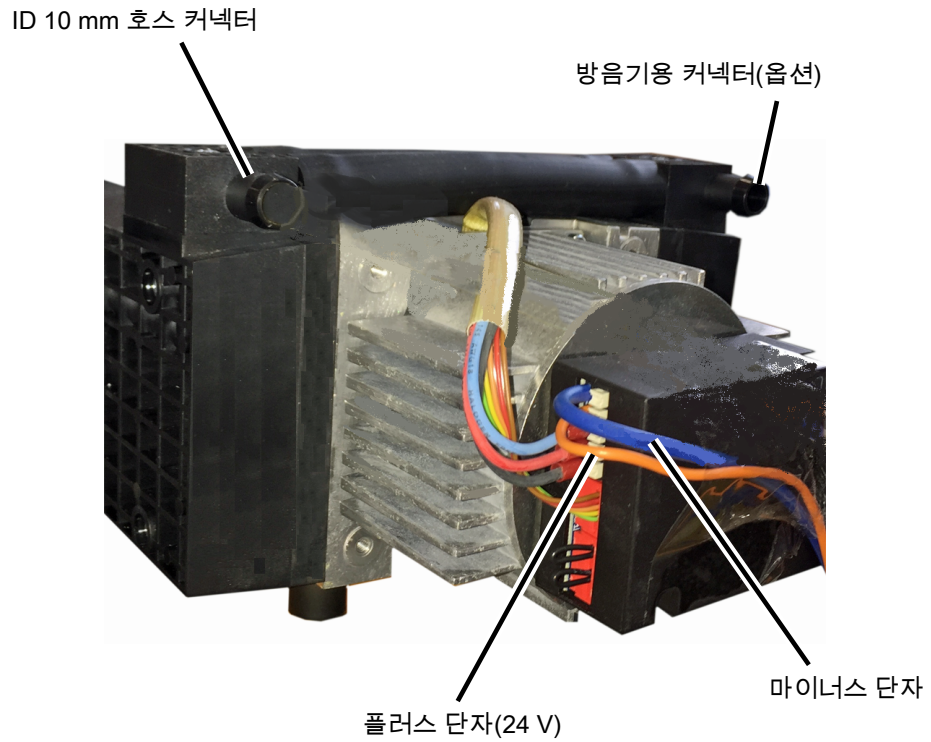
약어 4: INFICON 건식 포어 펌프
