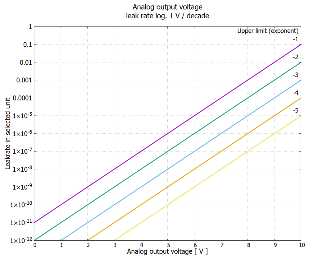
약어 12: 아날로그 출력 전압 누설률 대수 1V/디케이드
