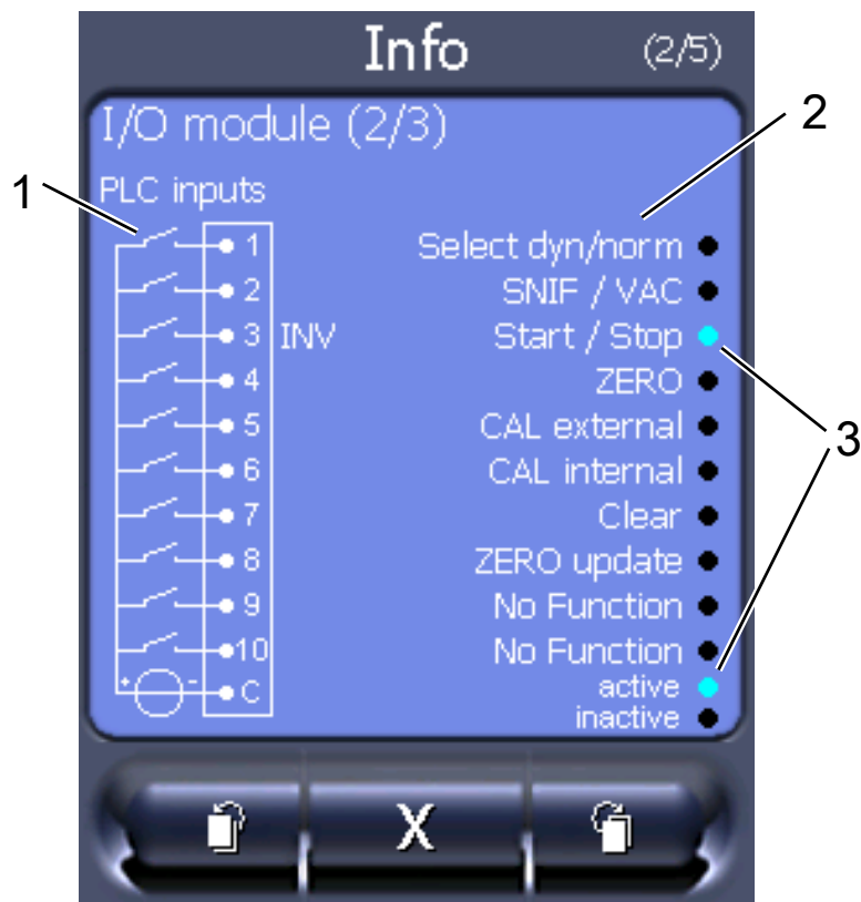
약어 15: I/O 모듈(2): 디지털 입력부 관련 시각화 정보
