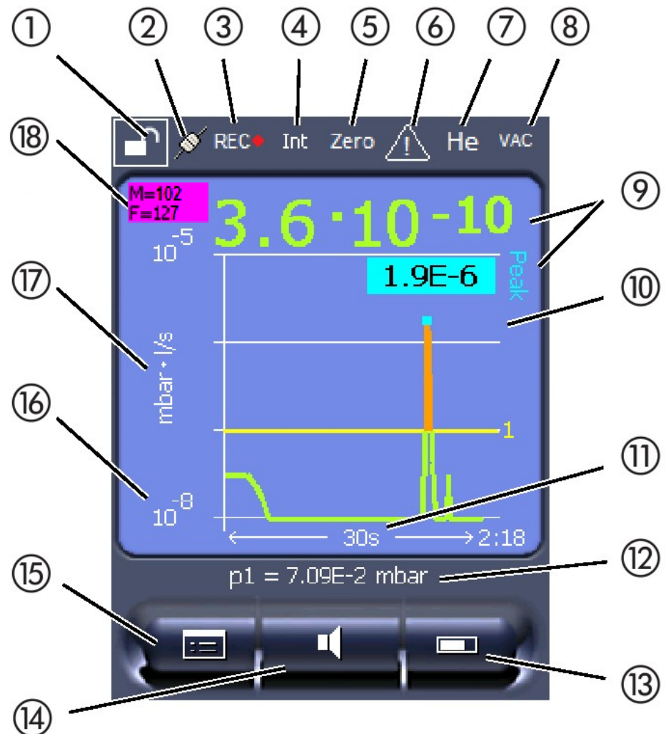
약어 14: 측정 디스플레이
