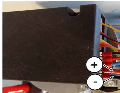
약어 10: INFICON 건식 포어 펌프에서의 단자판
