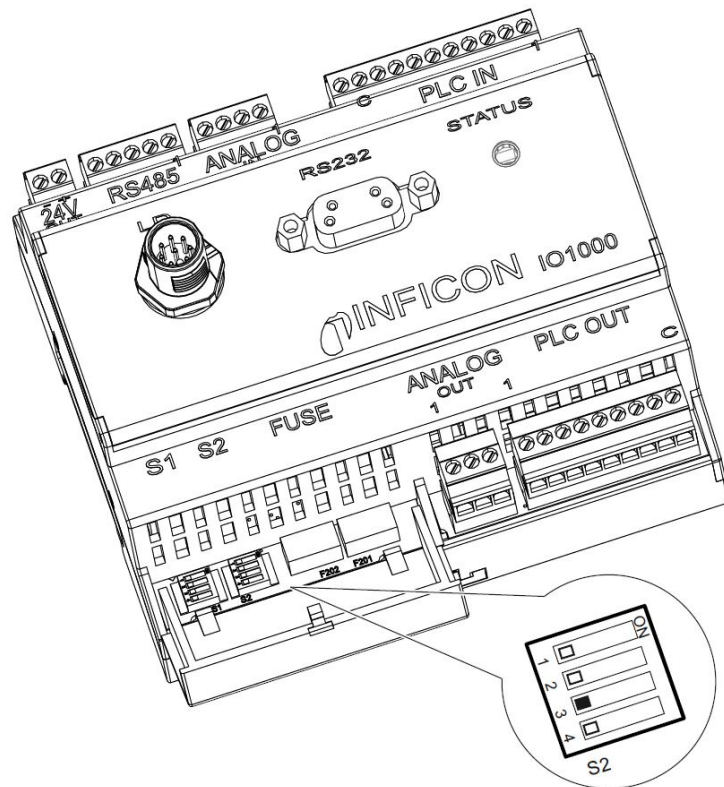
약어 19: I/O 모듈 DIP 스위치
