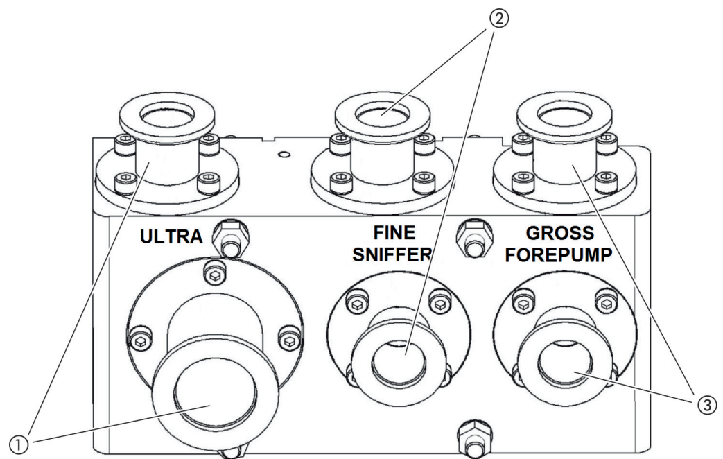
약어 5: 연결 블록
