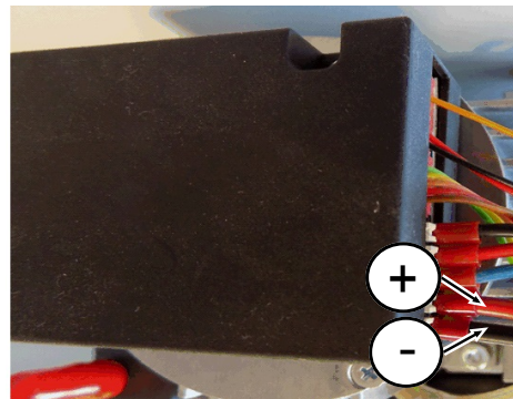
약어 9: INFICON 건식 포어 펌프에서의 단자판
