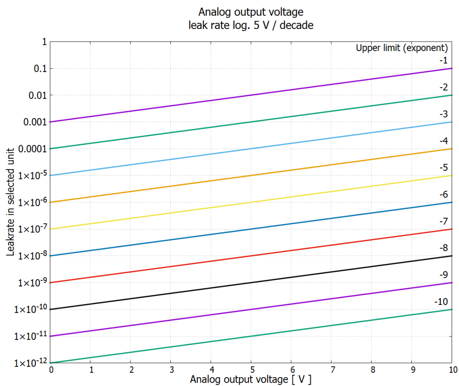
약어 13:아날로그 출력 전압 누설률 대수 5 V/디케이드
