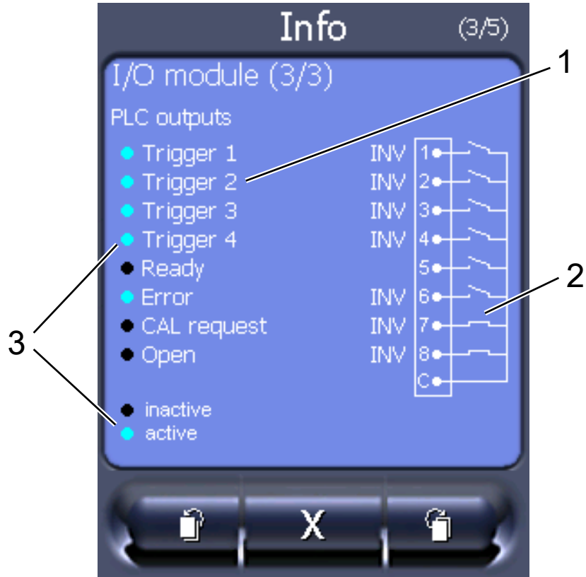
약어 16: 디지털 출력부 관련 시각화 정보
