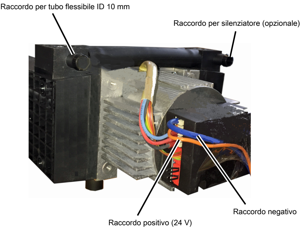
Fig. 4: Pre-pompa a secco di INFICON
