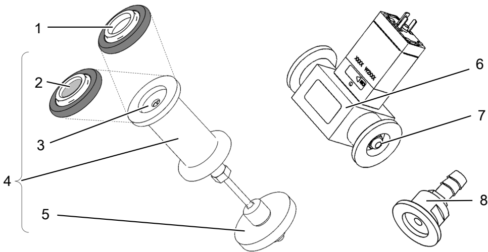
Fig. 23: Valvola a farfalla per AQ
