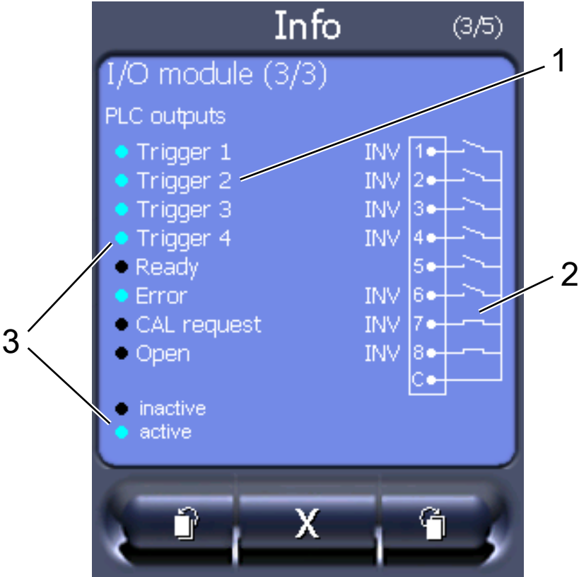
Fig. 16: Informazioni visualizzati sulle uscite digitali
