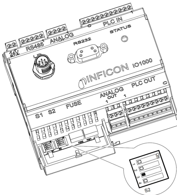
Fig. 19: Dip-switch del modulo I/O
