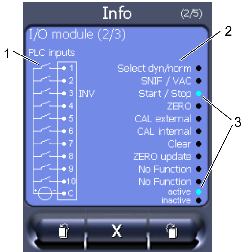
Fig. 15: Moduli I/O (2): Informazioni visualizzati sulle entrate digitali
