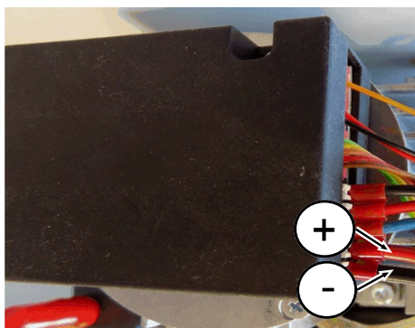
Fig. 9: Morsettiera sulla pre-pompa a secco INFICON
