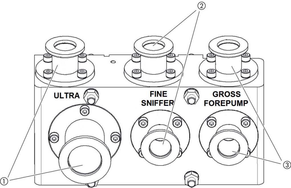
Fig. 5: Blocco di connessione
