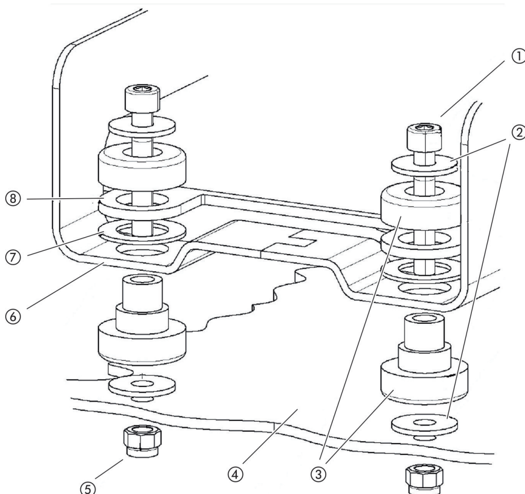
Fig. 8: Componenti di un elemento di fissaggio
