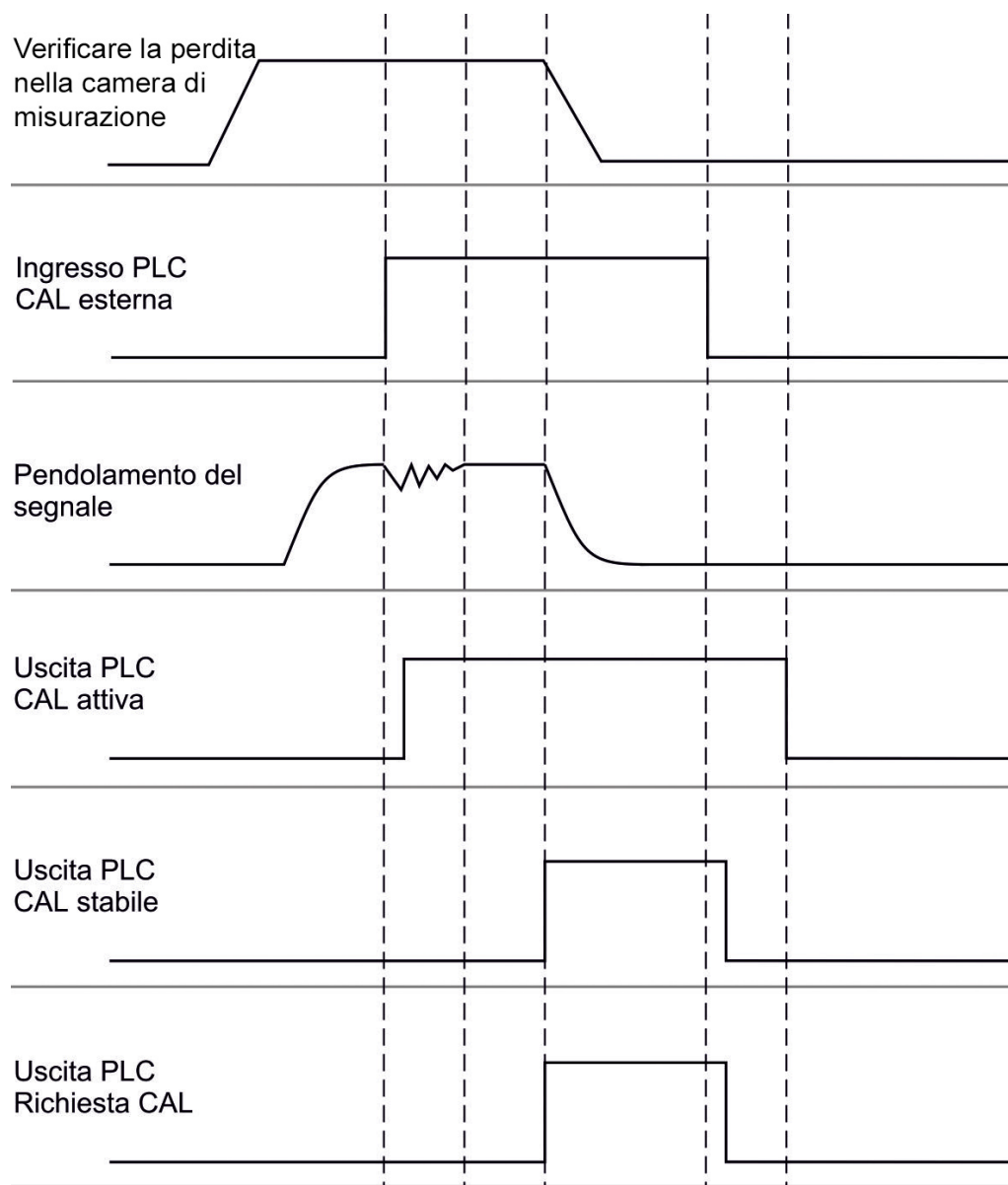
Fig. 11: Calibrazione esterna con IO1000 in un apparecchio per la modalità AQ. Descrizione degli ingressi e delle uscite PLC, vedere "Configurare gli ingressi e le uscite [► 53]"
