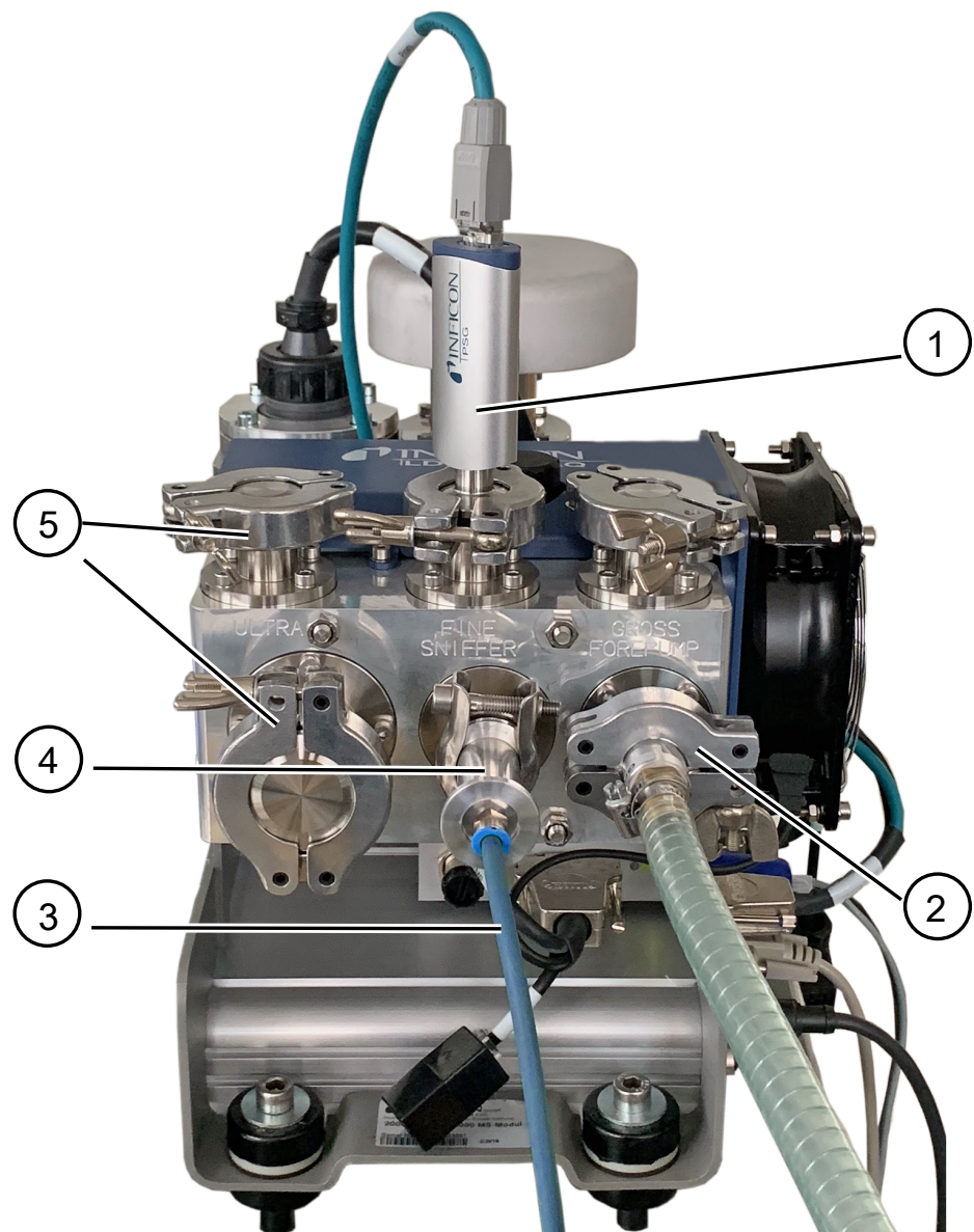
Fig. 2: Modulo spettrometro di massa (versione ad accumulo)
