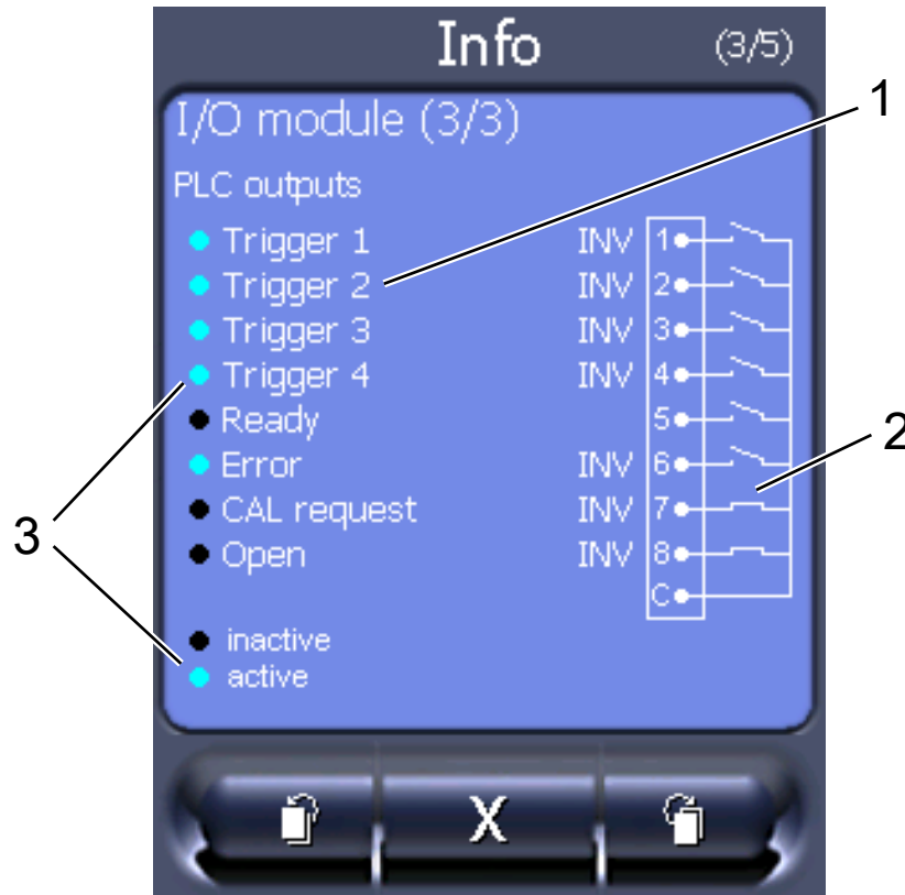
Abb. 16: Visualisierte Informationen zu den digitalen Ausgängen
