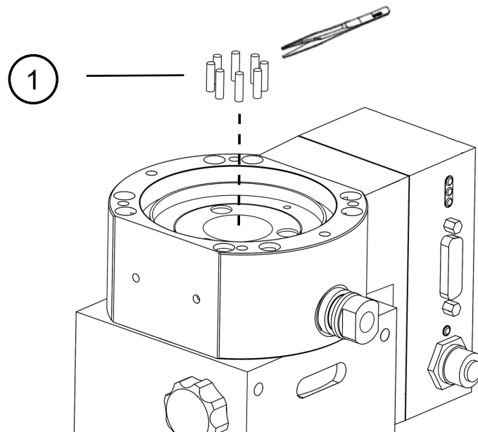
Abb. 21: Abbildung zeigt Modell A, Modell B analog
