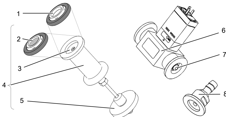
Abb. 23: Drossel für AQ
