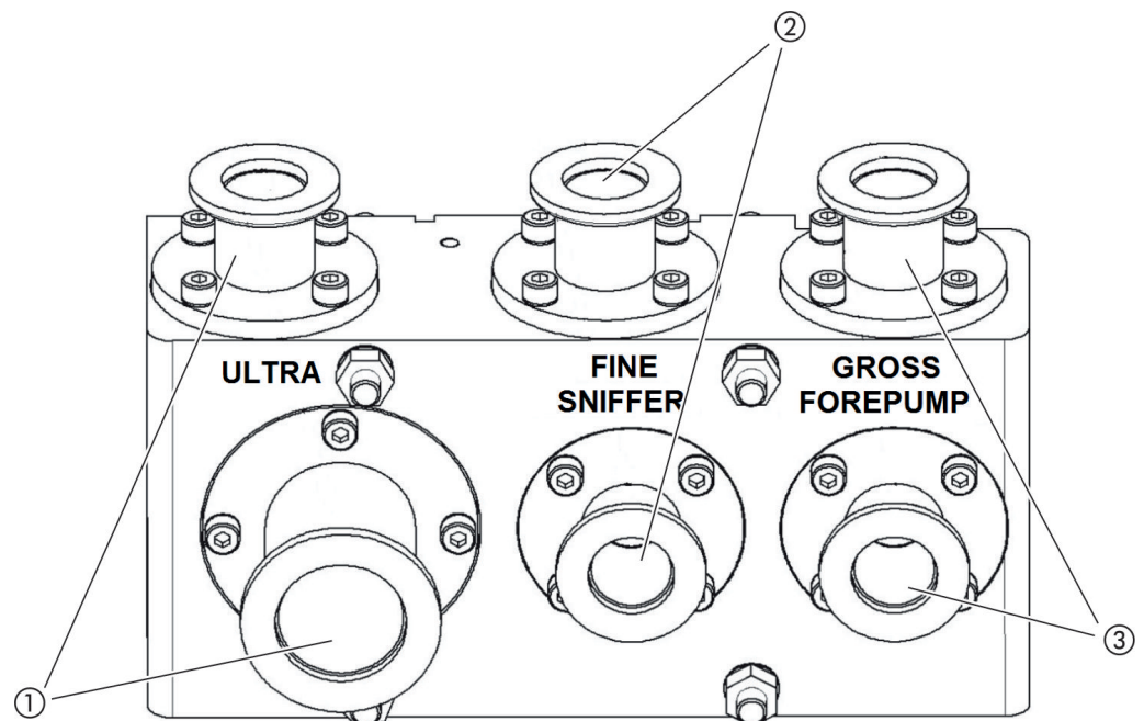
Abb. 5: Anschlussblock
