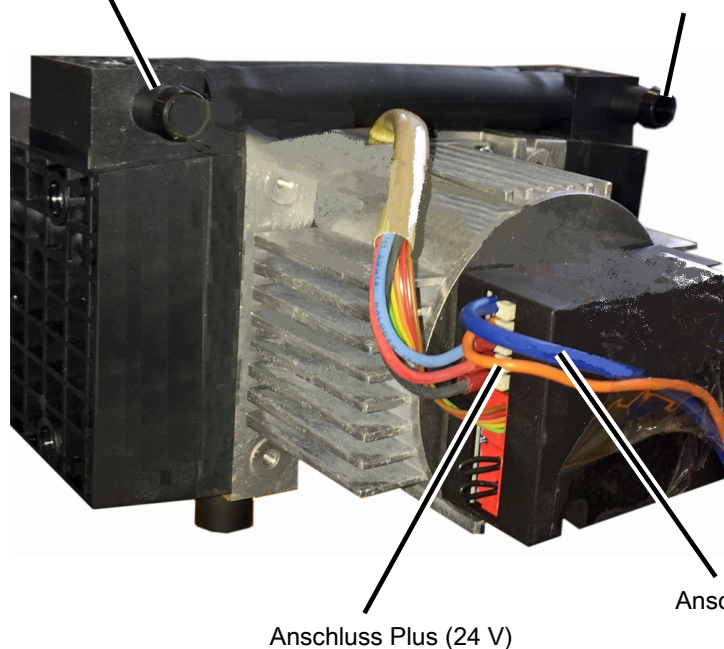
Abb. 4: Trockene Vorpumpe von INFICON
