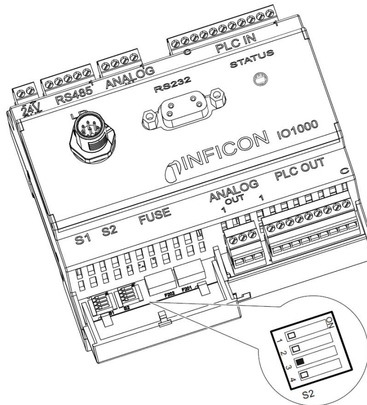
Abb. 19: DIP-Schalter am I/O-Modul
