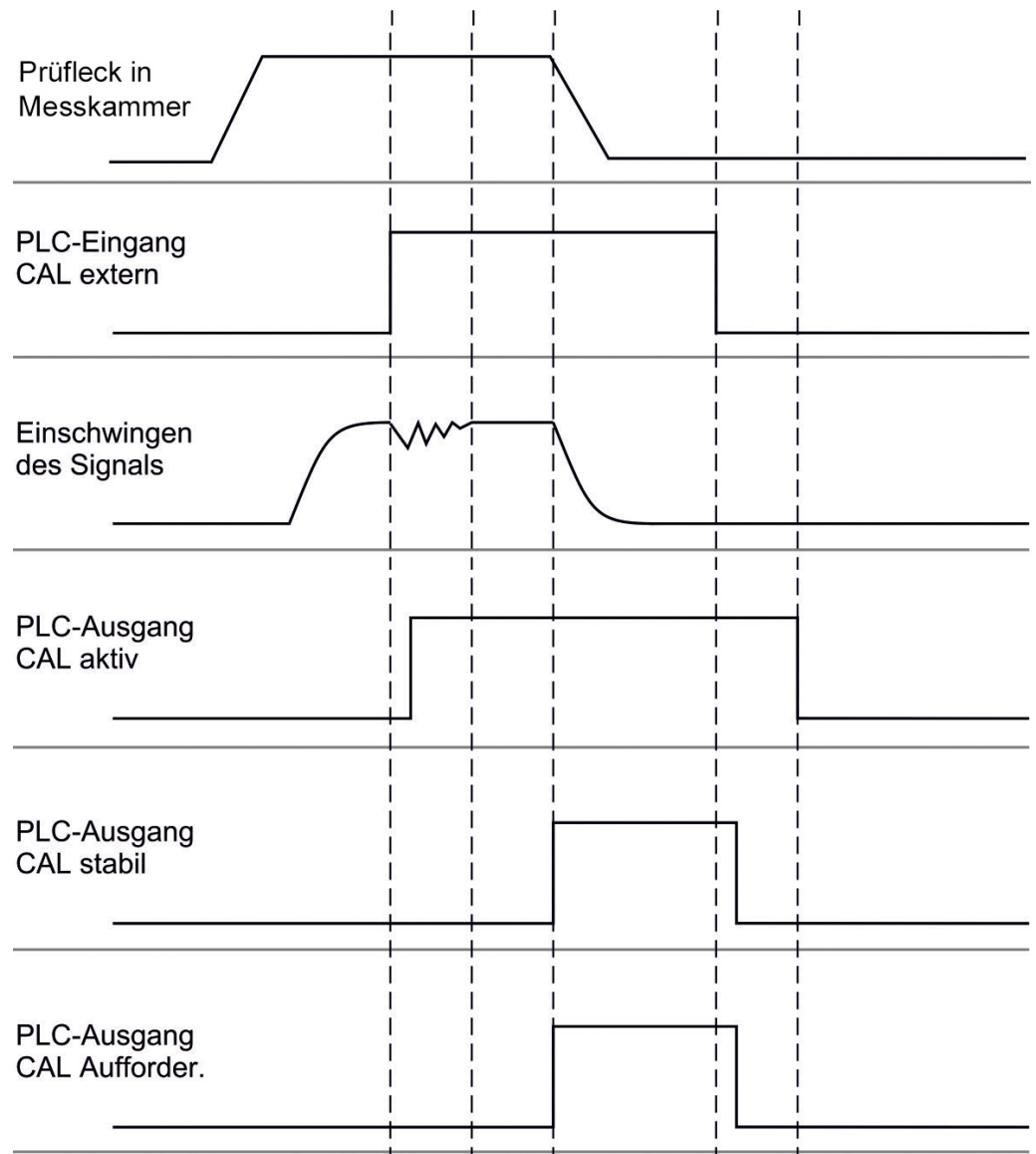
Abb. 11: Externes Kalibrieren mit IO1000 bei einem Gerät für den Modus AQ. Beschreibung der PLC-Ein- und Ausgänge siehe "Ein- und Ausgänge belegen [► 51]".
