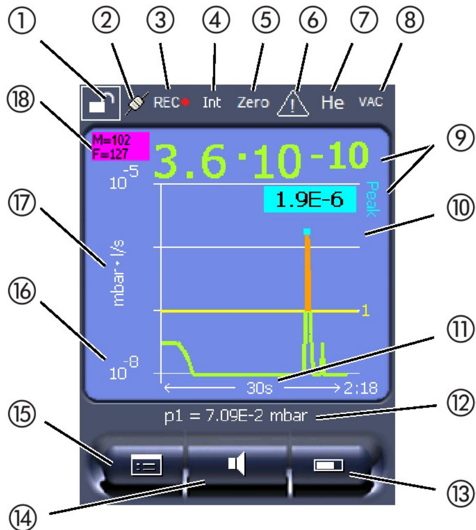
Abb. 14: Messanzeige
