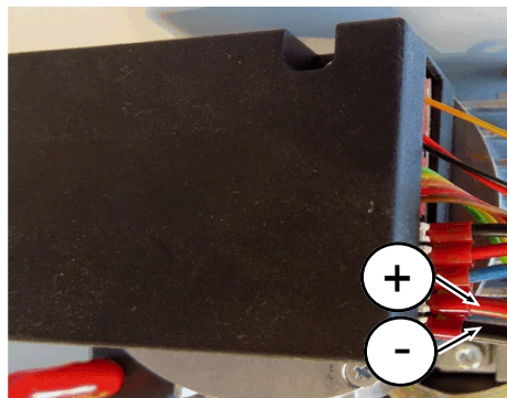
Abb. 10: Anschlussleiste an der trockenen Vorpumpe von INFICON
