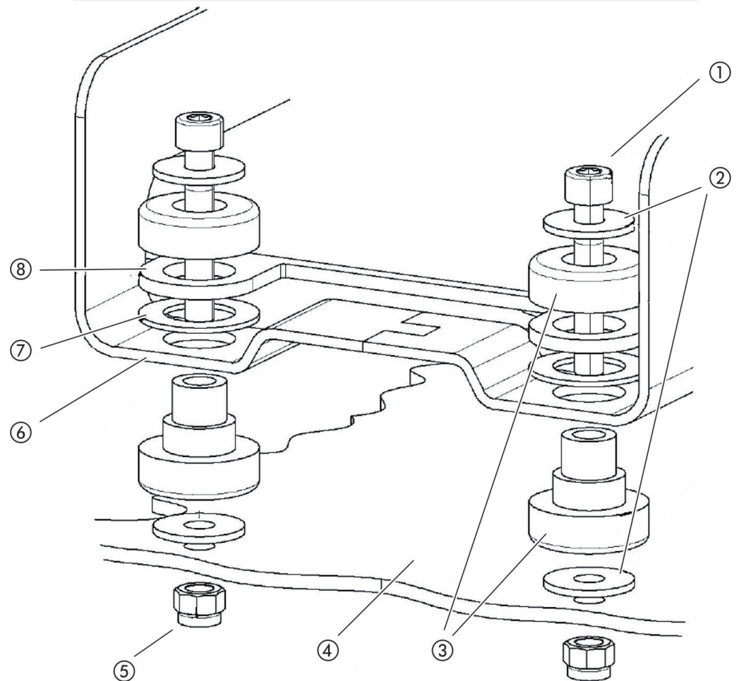
Abb. 8: Komponenten eines Befestigungselements
