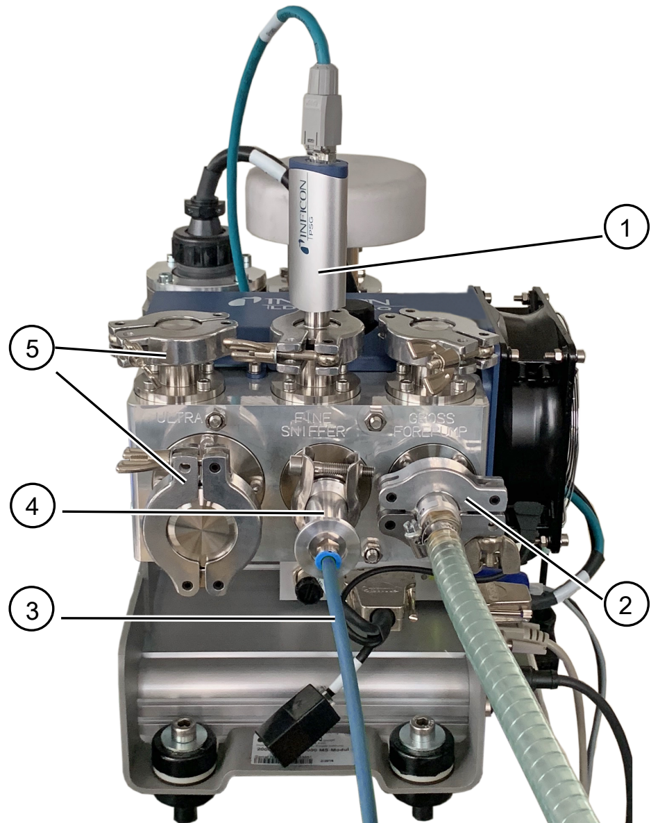
Abb. 2: Massenspektrometer-Modul (Ausführung Akkumulation)
