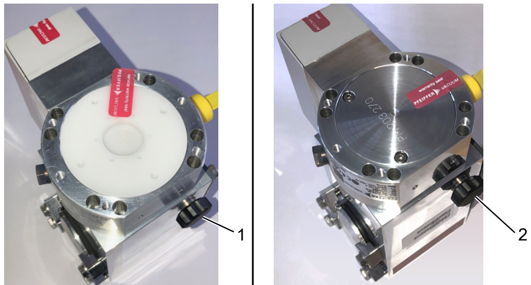
Abb. 20: Turbomolekularpumpe SplitFlow 80 mit unterschiedlichen Deckeln
