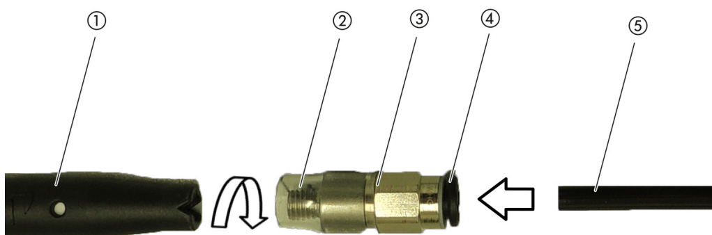
Fig. 5: Montaje del tubo flexible de prolongación
