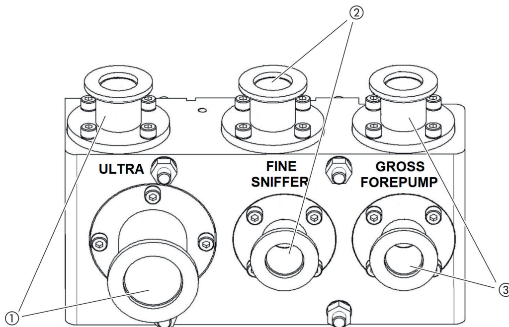
Obr. 2: Blok přípojů
