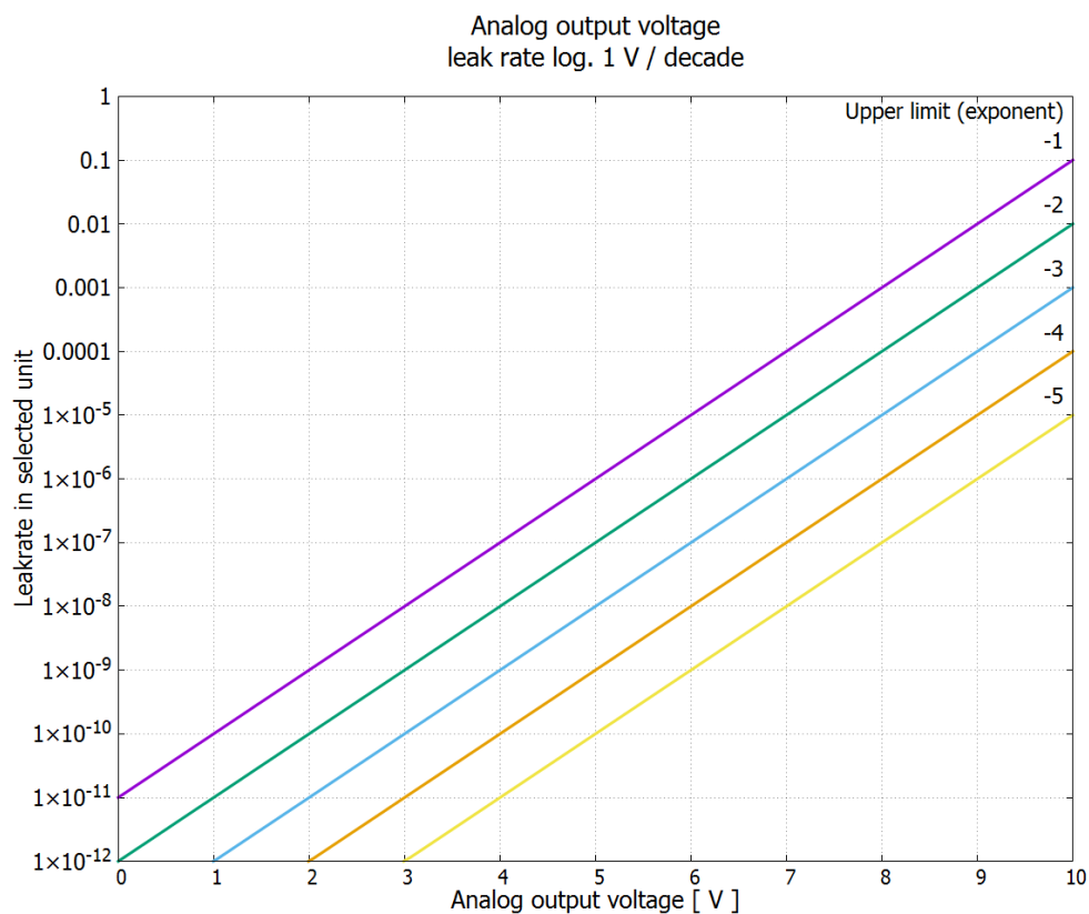
Obr. 9: Analogové výstupní napětí měří netěsnosti log. 1 V/dekáda
