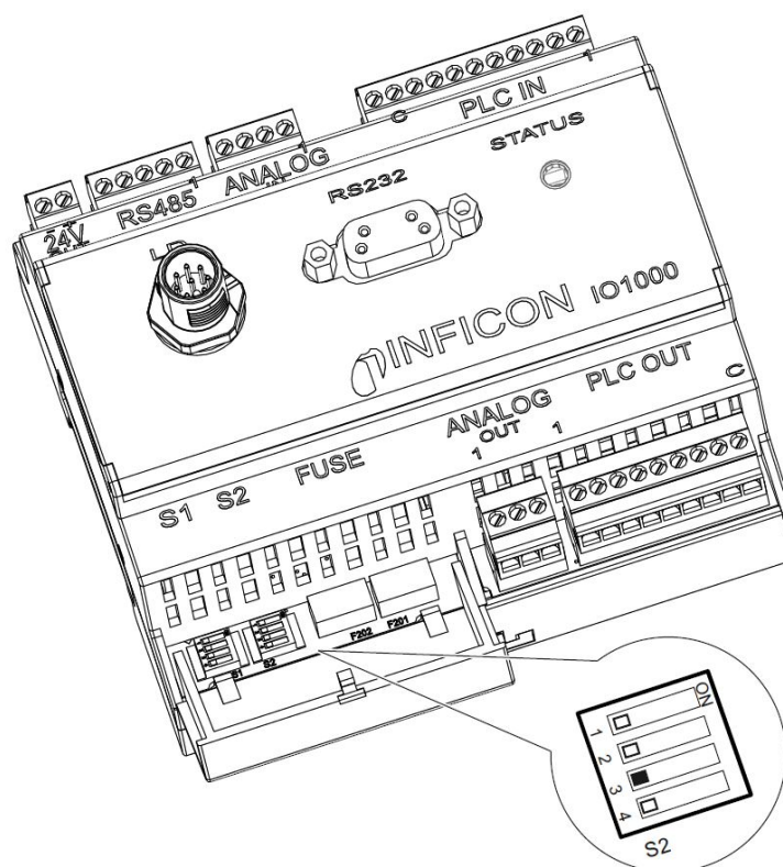
Obr. 16: DIP spínače na I/O modulu
