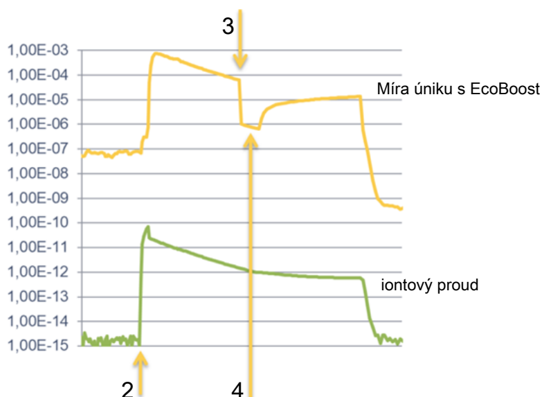
Obr. 8: Příklad křivek měření (EcoBoost)
