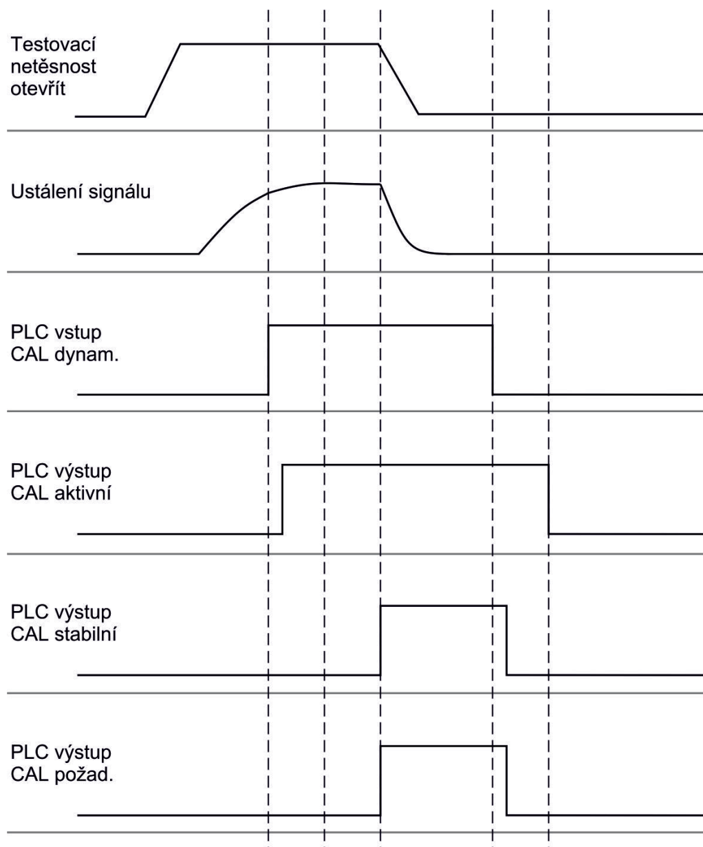
Obr. 7: Obr. 7 Externí dynamická kalibrace s IO1000 na příkladu vedení číhací sondy SL3000XL, popis vstupů a výstupů PLC: viz „Obsazení vstupů a výstupů [► 56]“
