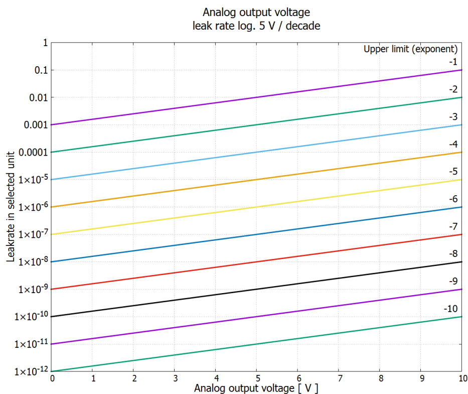
Obr. 10: Analogové výstupní napětí měří netěsnosti log. 5 V/dekáda
