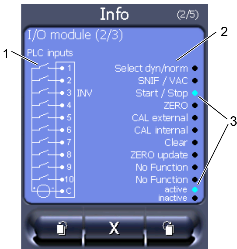
Obr. 12: I/O moduly (2): Vizualizované informace k digitálním vstupům
