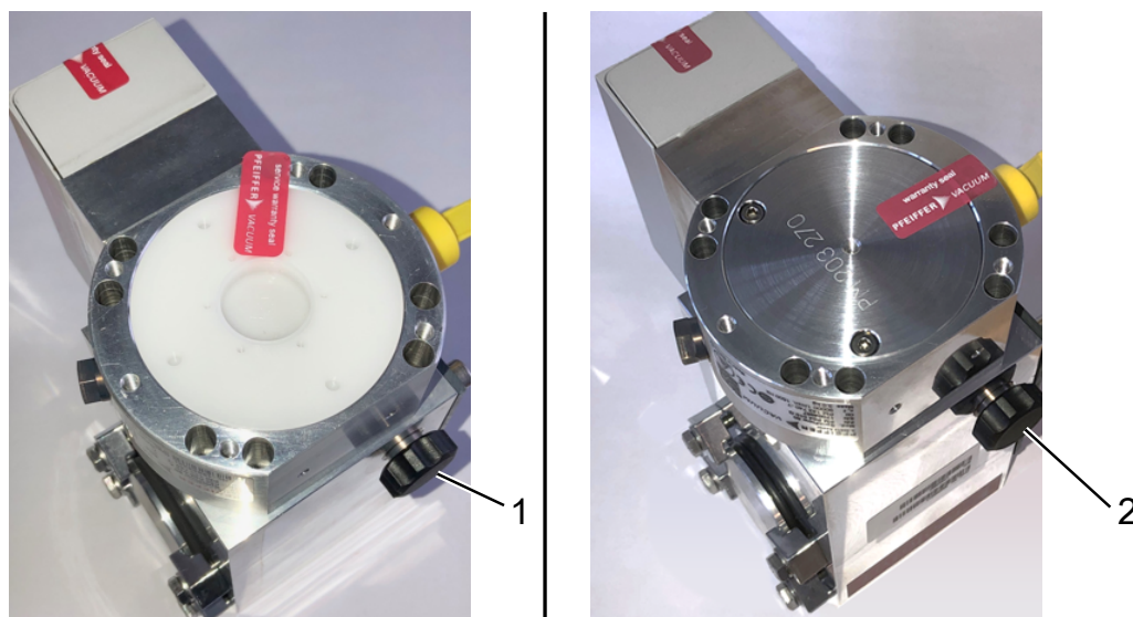
Obr. 17: Turbomolekulární vývěva SplitFlow 80 s různými víky
