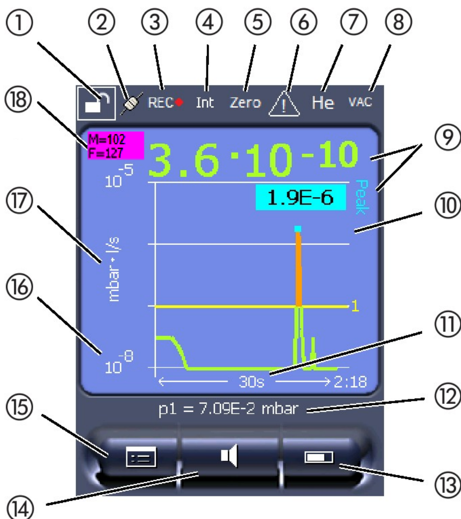
Obr. 11: Zobrazení měření
