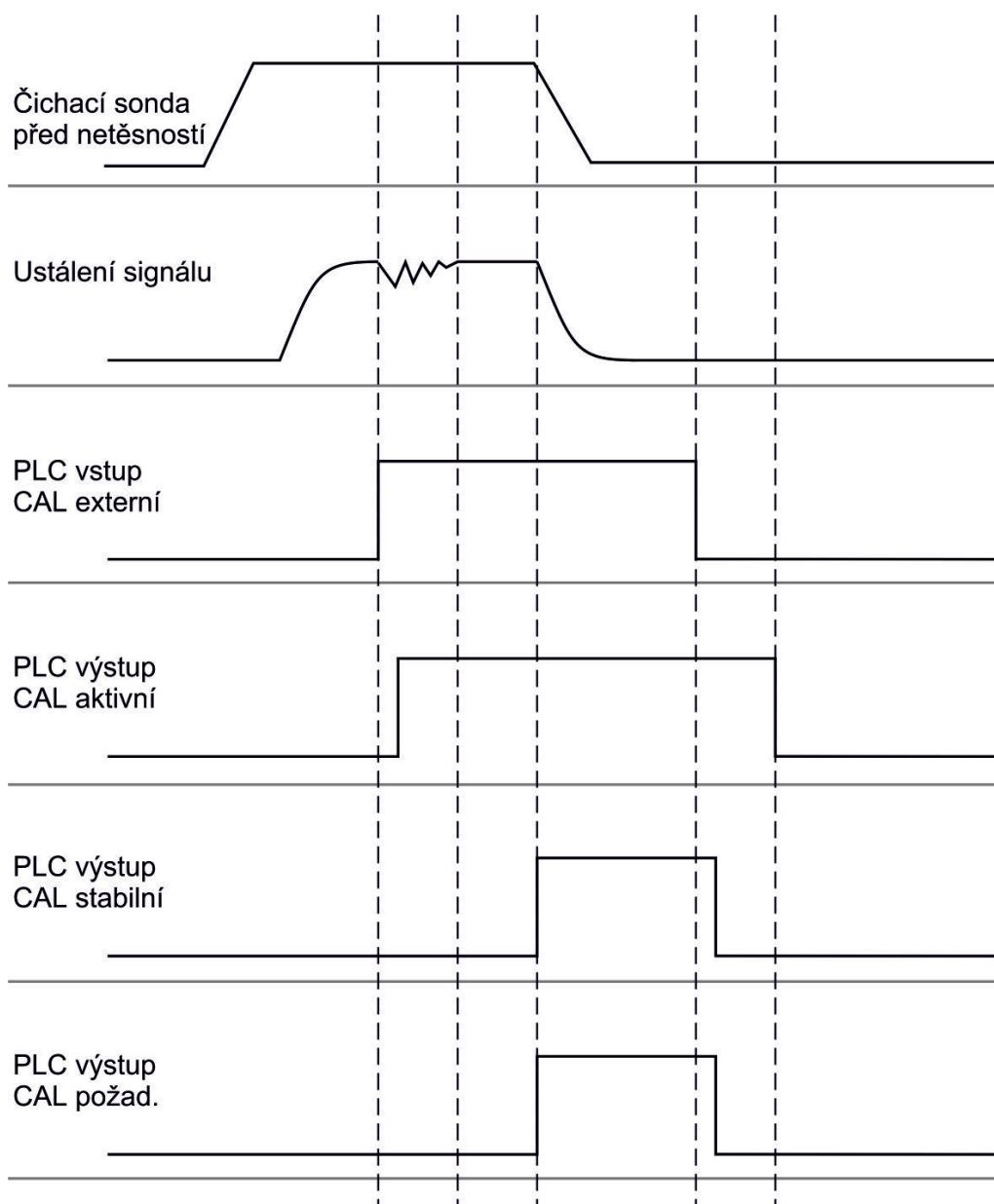
Obr. 6: Externí kalibrace s IO1000 na příkladu vedení číhací sondy SL3000XL, popis vstupů a výstupů PLC: viz „Obsazení vstupů a výstupů [► 56]“
