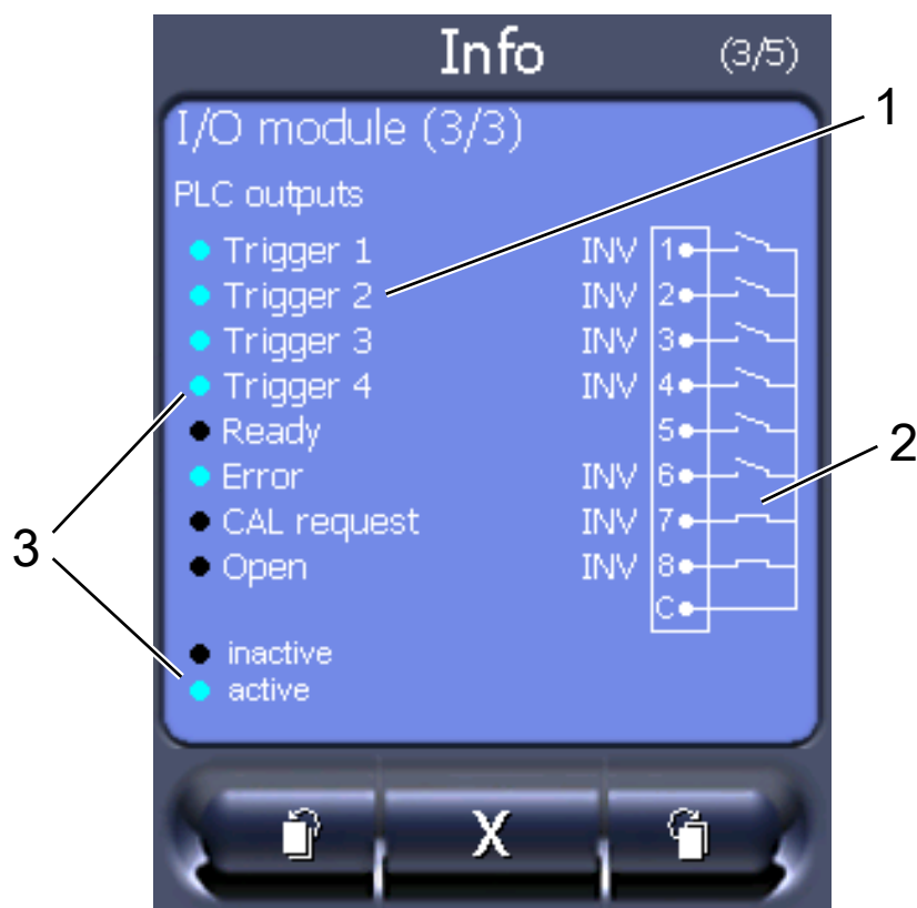
Obr. 13: Vizualizované informace k digitálním výstupům
