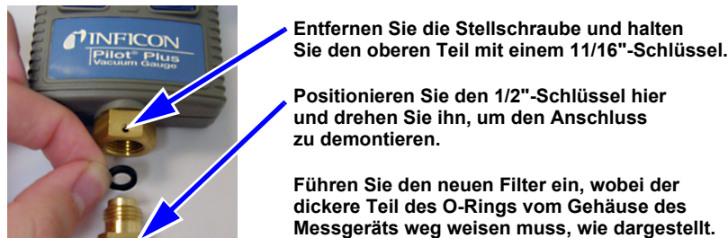
Abbildung 5. Pilot Plus-Anschluss
